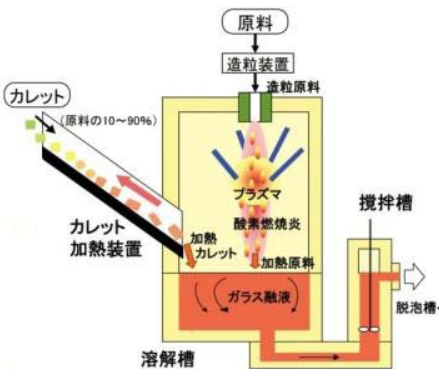
プラズマによる革新的ガラス製造システム
