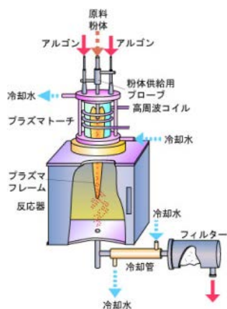
RF プラズマによる ナノ粒子合成装置
